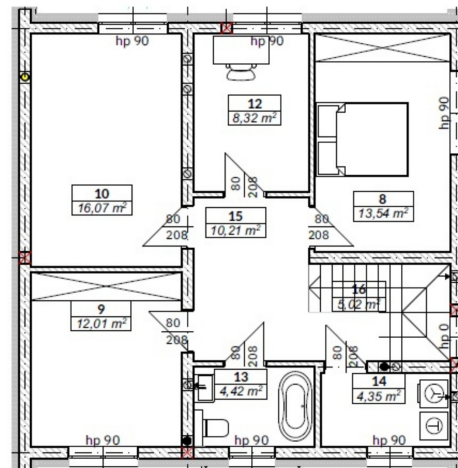
RZUT PIĘTRA
