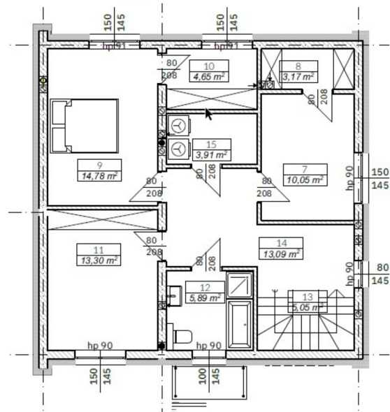
RZUT PIĘTRA
