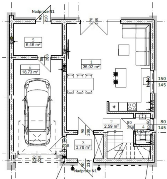
RZUT PARTERU
